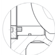
Металлическое уплотнение тип В
