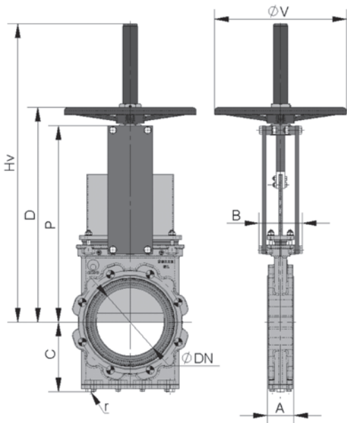
Размеры затворов с ручным приводом (не выдвигной шток)
