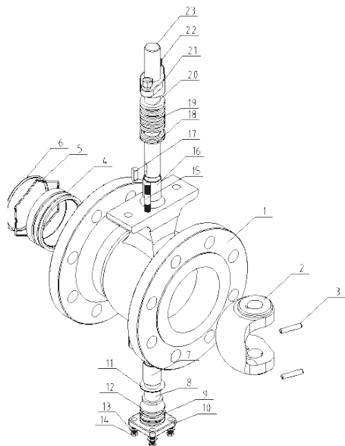
Металлическое уплотнение тип А
